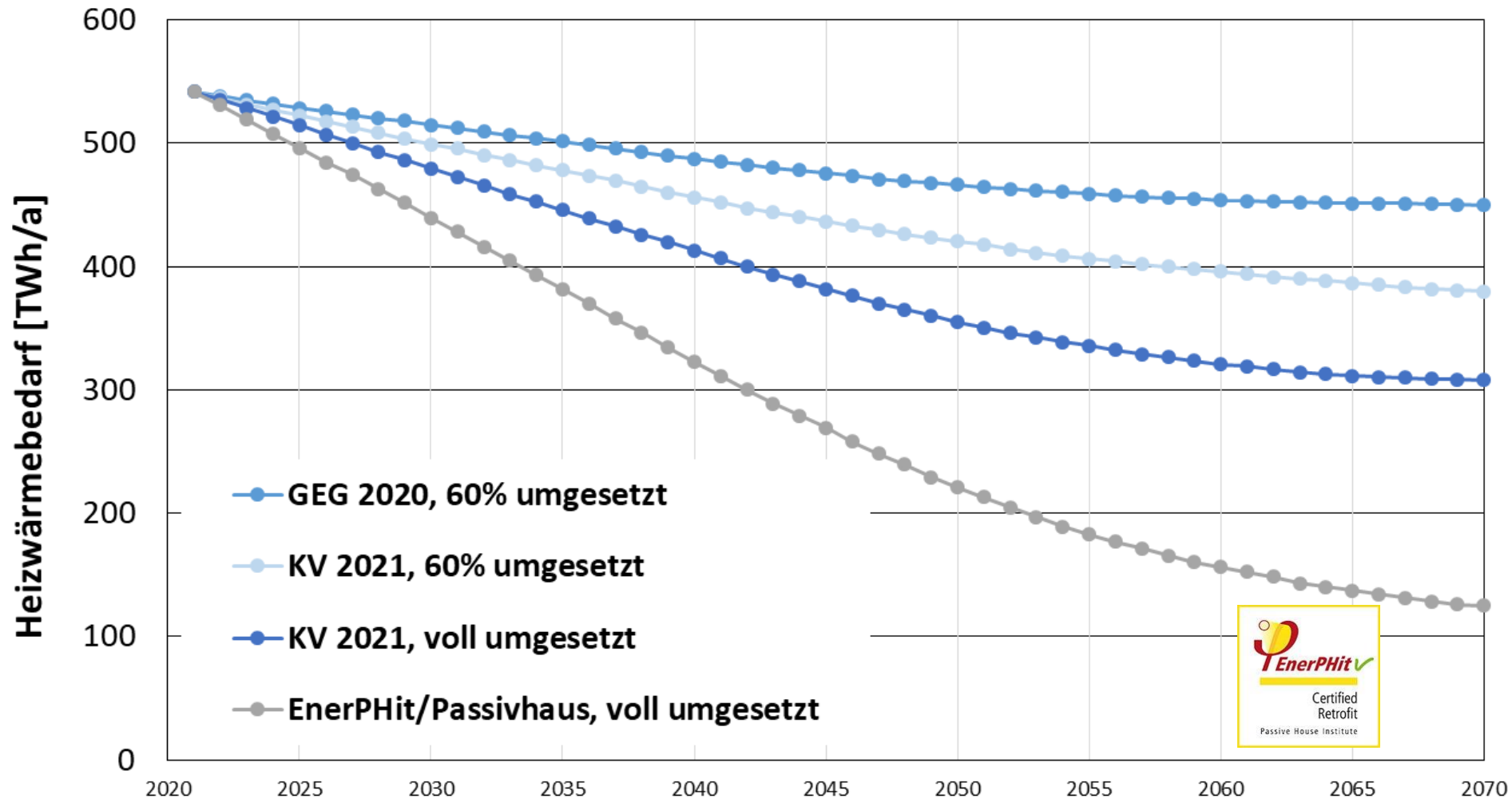
Heizwärmebedarf
