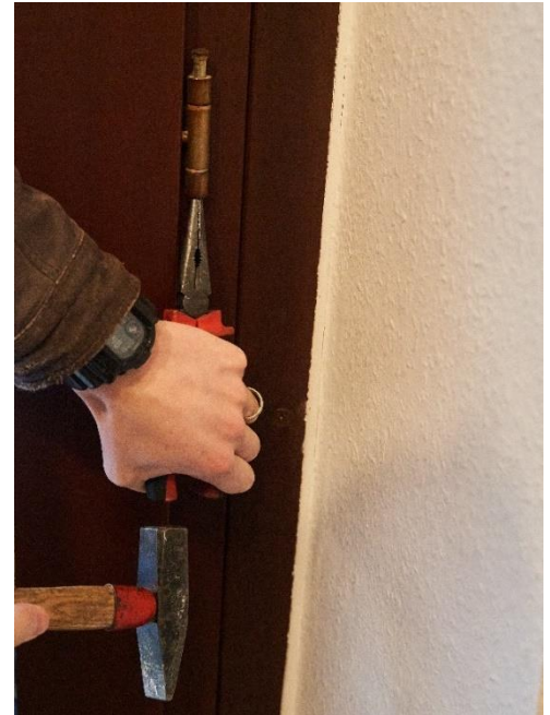
Abbildung 9: Ausrücken des Bolzens aus den Angeln
